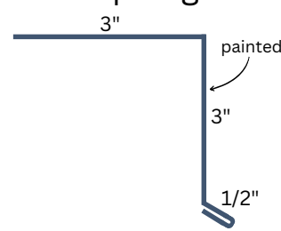
Drip Edge
