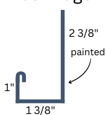
Door Edge
